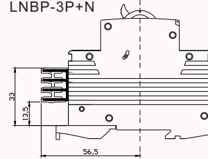
LNBP-3P+N
